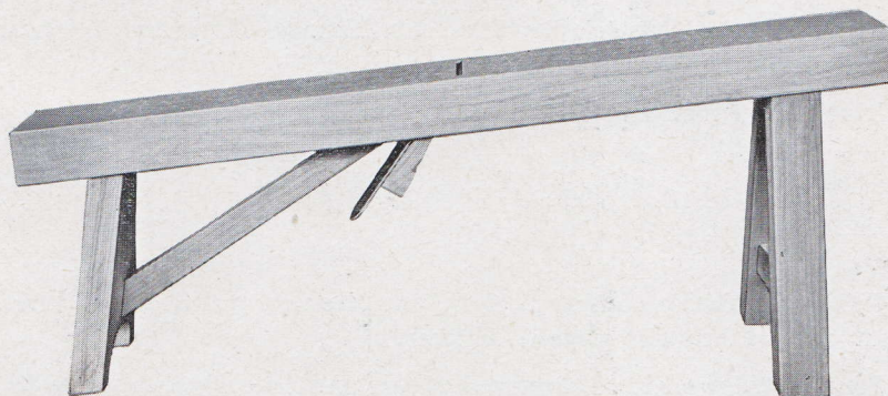
N° 280 COLOMBE DE TONNELIER
